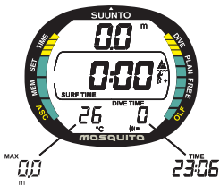
Fig. 3.4 Puesta en marcha III. Pantalla modo Superficie. La profundidad y el tiempo de inmersión están a cero. Presionando los botones +/- la pantalla muestra alternativamente la profundidad máxima y la hora.
