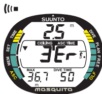
Fig. 3.20 Inmersión con paradas de descompresión, por encima de la profundidad techo. Aparecen la flecha hacia abajo y la mención Er. La alarma sonora se dispara igualmente.
