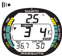
Fig. 3.14 Parada de Seguridad Obligatoria no respetada. La flecha hacia abajo y la alarma sonora le informan de que hace falta descender a la profundidad indicada por la mención CEILING.
