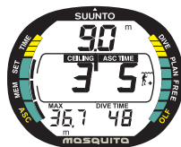
Fig. 3.18 Inmersión con paradas de descompresión por encima de la profundidad suelo. La flecha ha desaparecido y la mención ASC TIME no parpadea. Usted está en la zona de descompresión.
