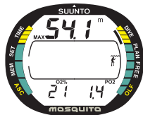
Fig. 3.21 Pantalla Nitrox. La profundidad máxima calculada en función del % O_2 (21%) y de la PO_2 (1,4 bar) es de 54,1 m.
